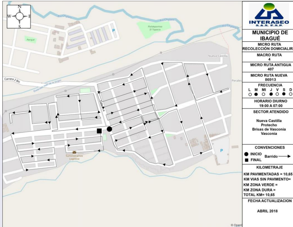
Ilustración 1. representación gráfica de micro ruta de recolección. febrero 2022
